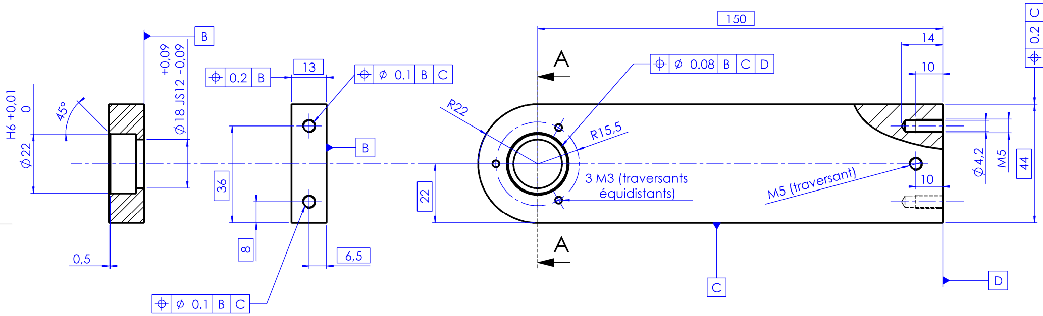
COUPE A-A
